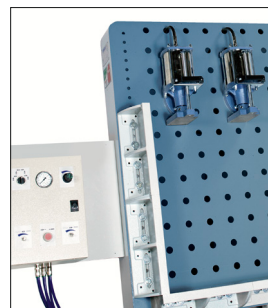
Comando bimanuale con gestione a 2 stazioni indipendenti.
